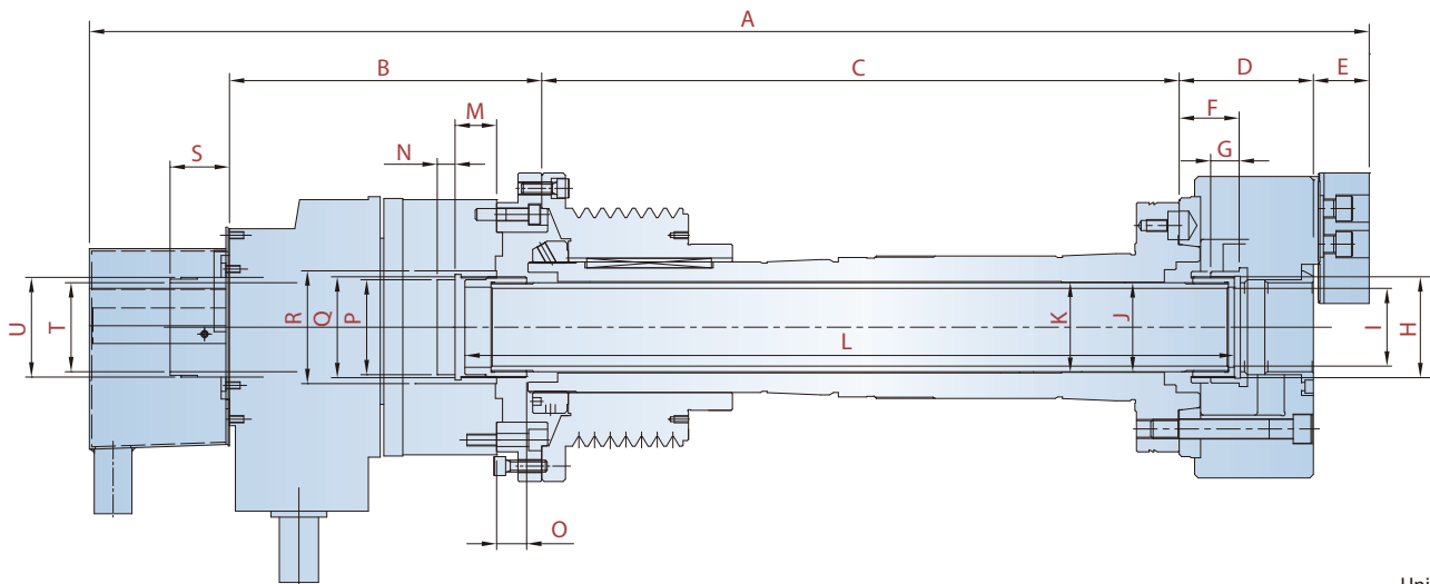
【 Spindle Dimension Drawing 】
